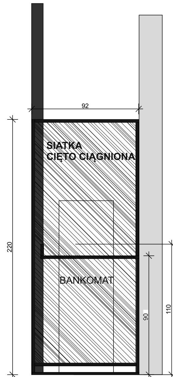
PRZEKRÓJ Z TYŁU
