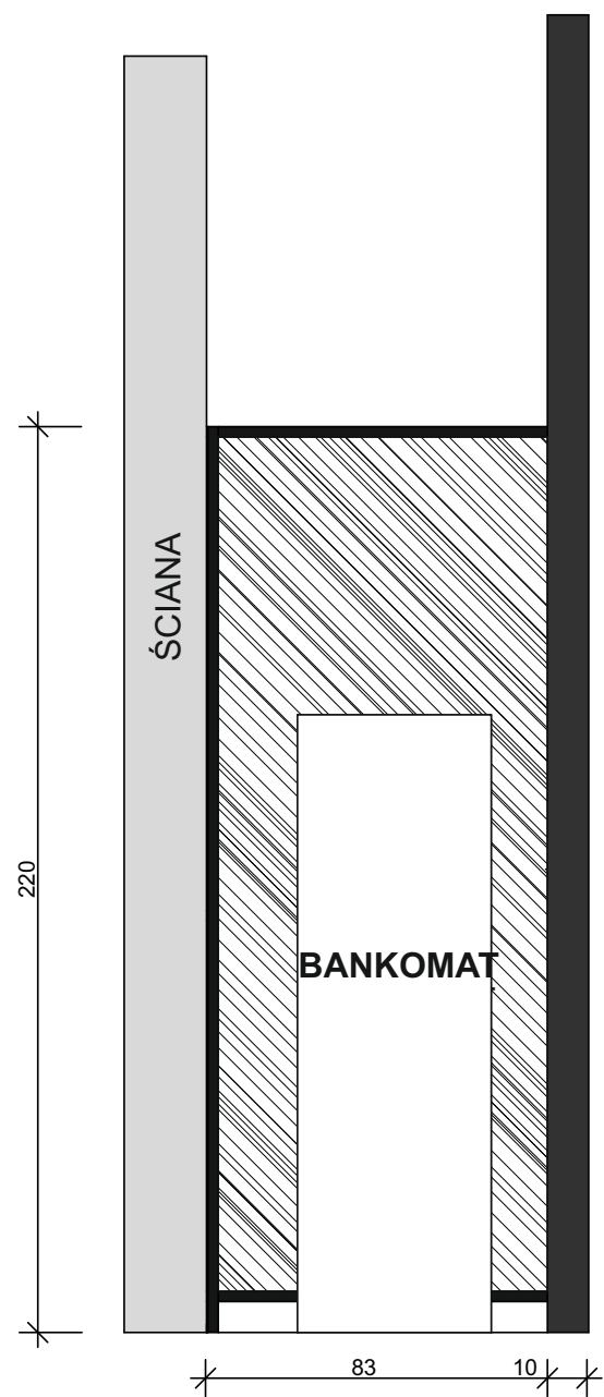
PRZEKRÓJ Z PRZODU OD KORYTARZA
